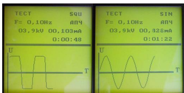
Рис.1. Показания дисплея во время работы
