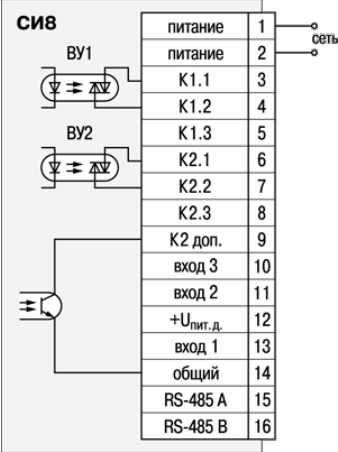
Схема подключения прибора СИ8 с оптосимисторным выходом (выход С)
