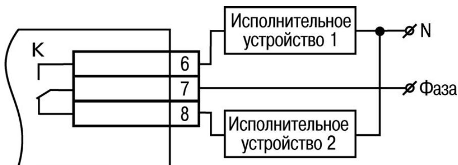
Схема подключения нагрузки к ВУ типа Р
