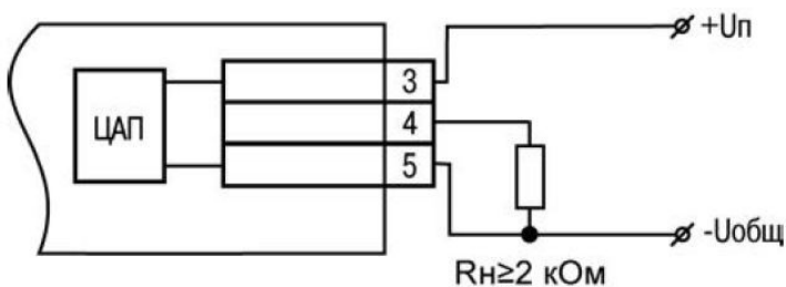
Пример подключения ВУ типа У
