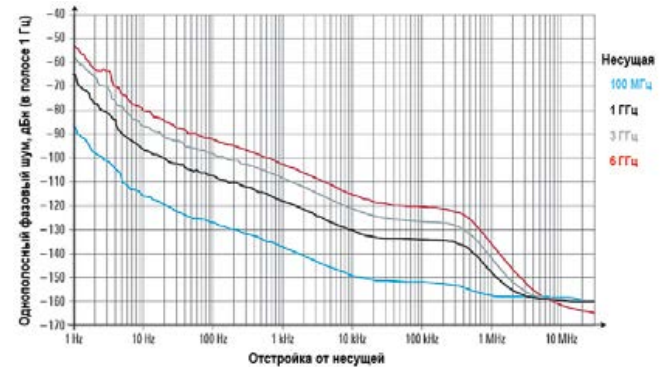
Измеренные значения фазового шума с опцией SMBVB-B1H
