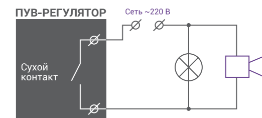
Схема подключения внешнего устройства для подачи звукового (светового) сигнала.
