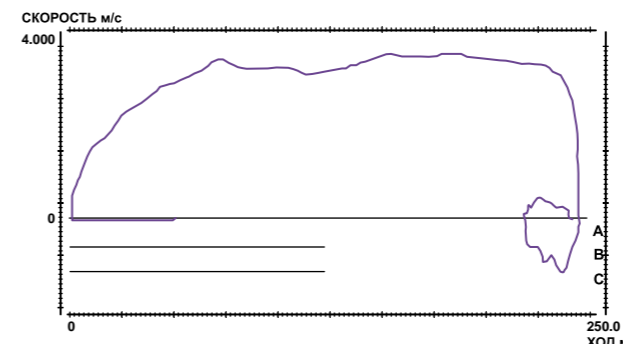
График зависимости скорости от хода
