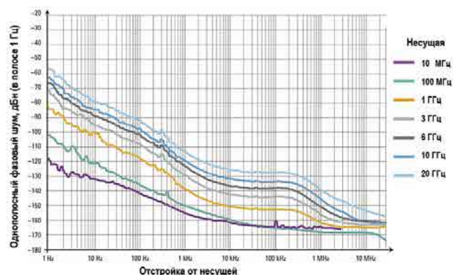
Измеренные значения фазового шума с опцией R&S®SMAB-B711
