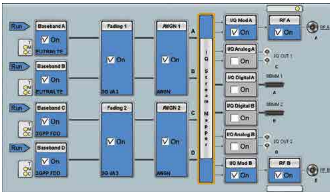
Блок-схема генератора R&S®SMW200A, настроенного на одновременную генерацию сигнала двоянной соты стандарта HSPA и 2x2 ММО для LTE с коррелированными каналами замираний
