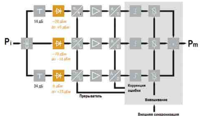
Архитектура 3-канального датчика
