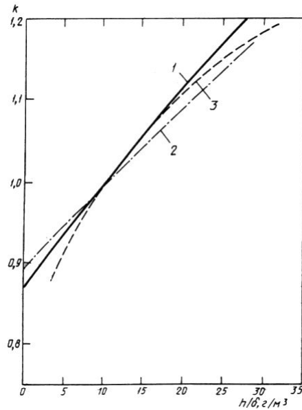
1 - переменное напряжение; 2 - импульс напряжения; 3 - постоянное напряжение
