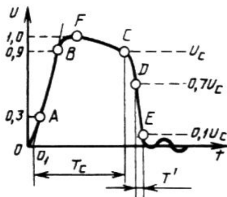
Рисунок 9 - Грозовой импульс, срезанный на спаде импульса
