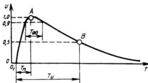
Рисунок 13 - Апериодический коммутационный импульс
