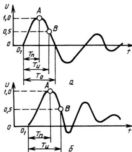
Рисунок 14 - Колебательный коммутационный импульс
