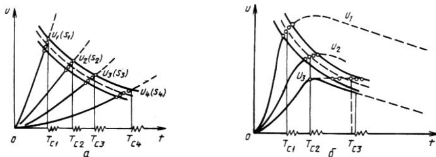
Рисунок 12 - Вольт-секундные характеристики
