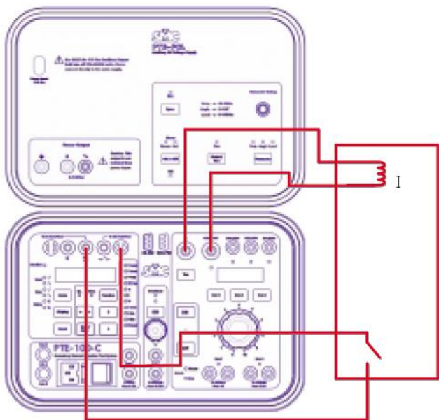
Проверка реле максимального тока
