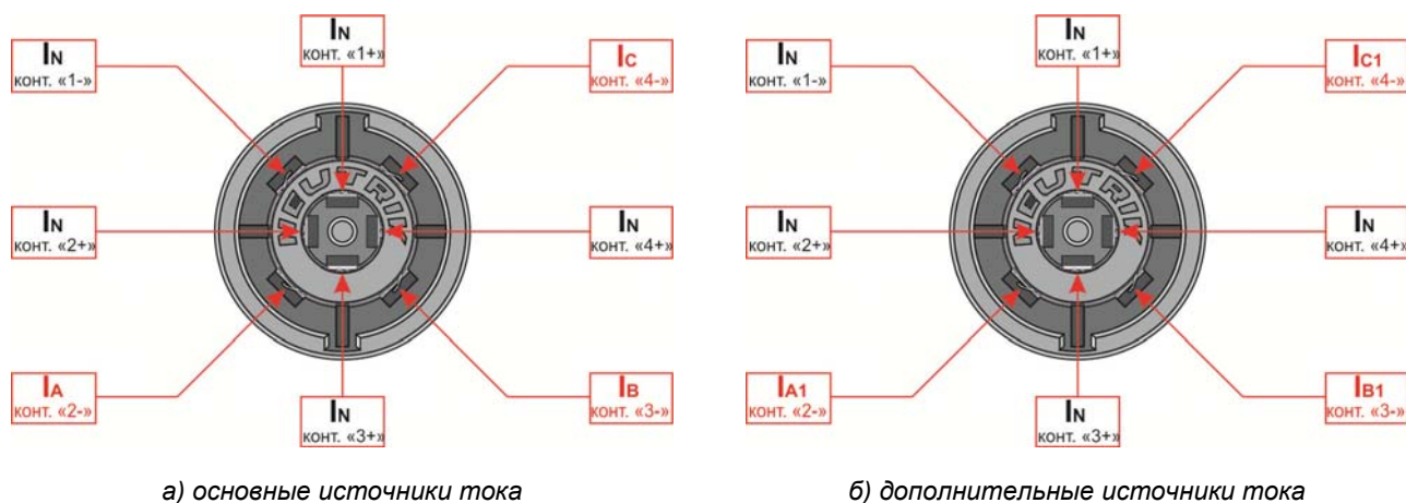
Рисунок 8.5 – Разъемы для подключения силовых кабелей тока
