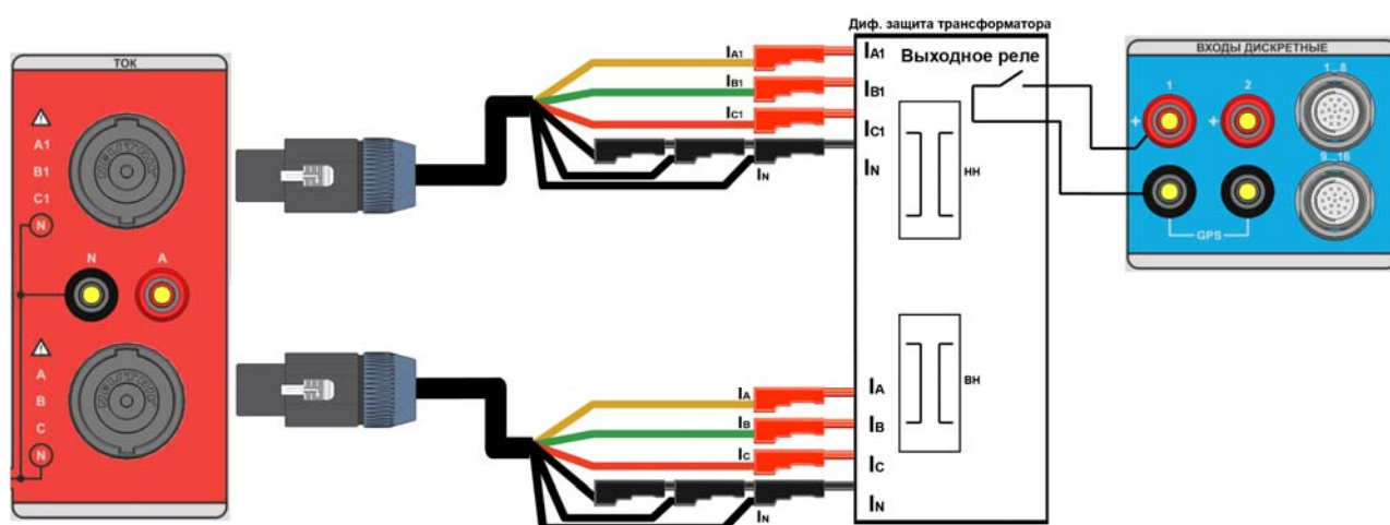
Рисунок 9.2 – Пример подключения дифференциальной защиты двухобмоточного трансформатора к РЕТОМ-61
