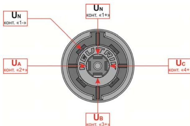
Рисунок 8.6 – Разъем для подключения силового кабеля напряжения
