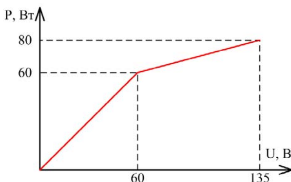
Рисунок 8.7 – Нагрузочная характеристика усилителей напряжения
