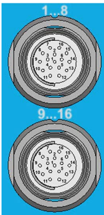
Рисунок 8.8 – Разъем для подключения к дискретным входам кабелей информационных КИ-04 (вид со стороны лицевой панели)
