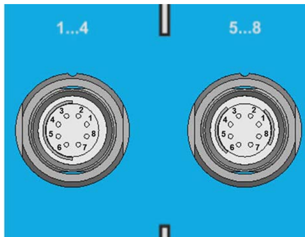
Рисунок 8.11 – Разъем для подключения к дискретным выходам кабелей коммутации КК-04-1, КК-04-2 БЫСТРЫЕ (вид со стороны лицевой панели)
