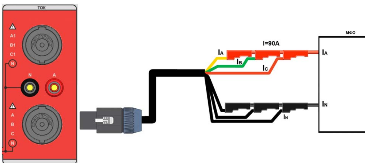
Рисунок 9.3 – Однофазное подключение токовых цепей
