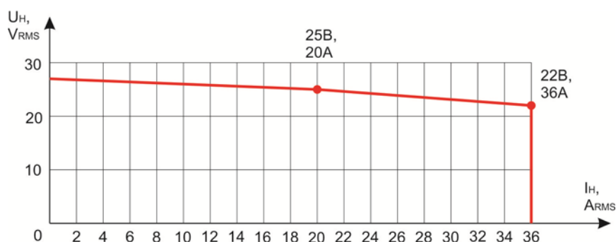
Рисунок 8.2 – Характеристика предельных режимов каналов тока
