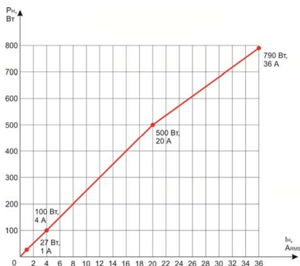
Рисунок 8.3 – Нагрузочная характеристика усилителей тока
