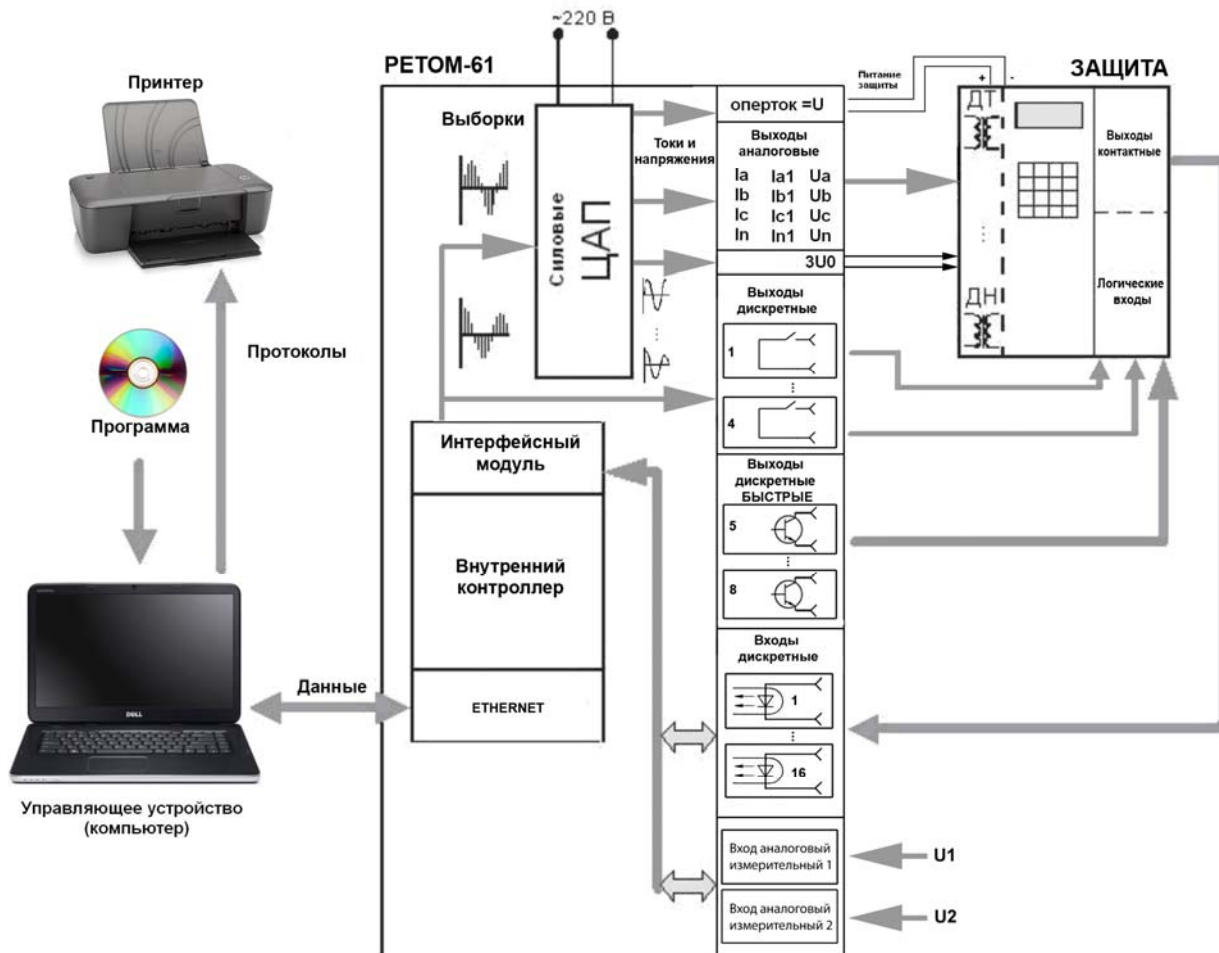
Рисунок 7.1 – Структура комплекса PETOM-61
