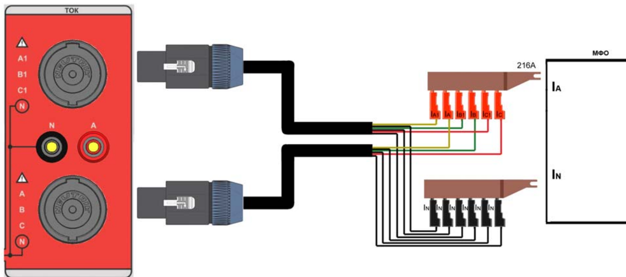
Рисунок 9.4 – Использование объединяющего устройства для тока более 100 А
