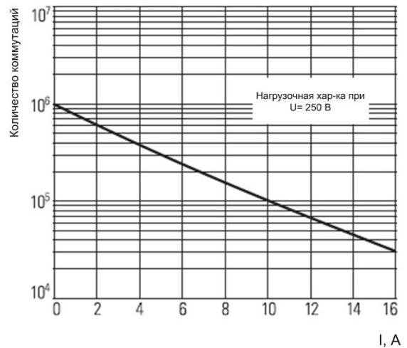
Рисунок 8.10 – Коммутационная износостойкость выходных реле
