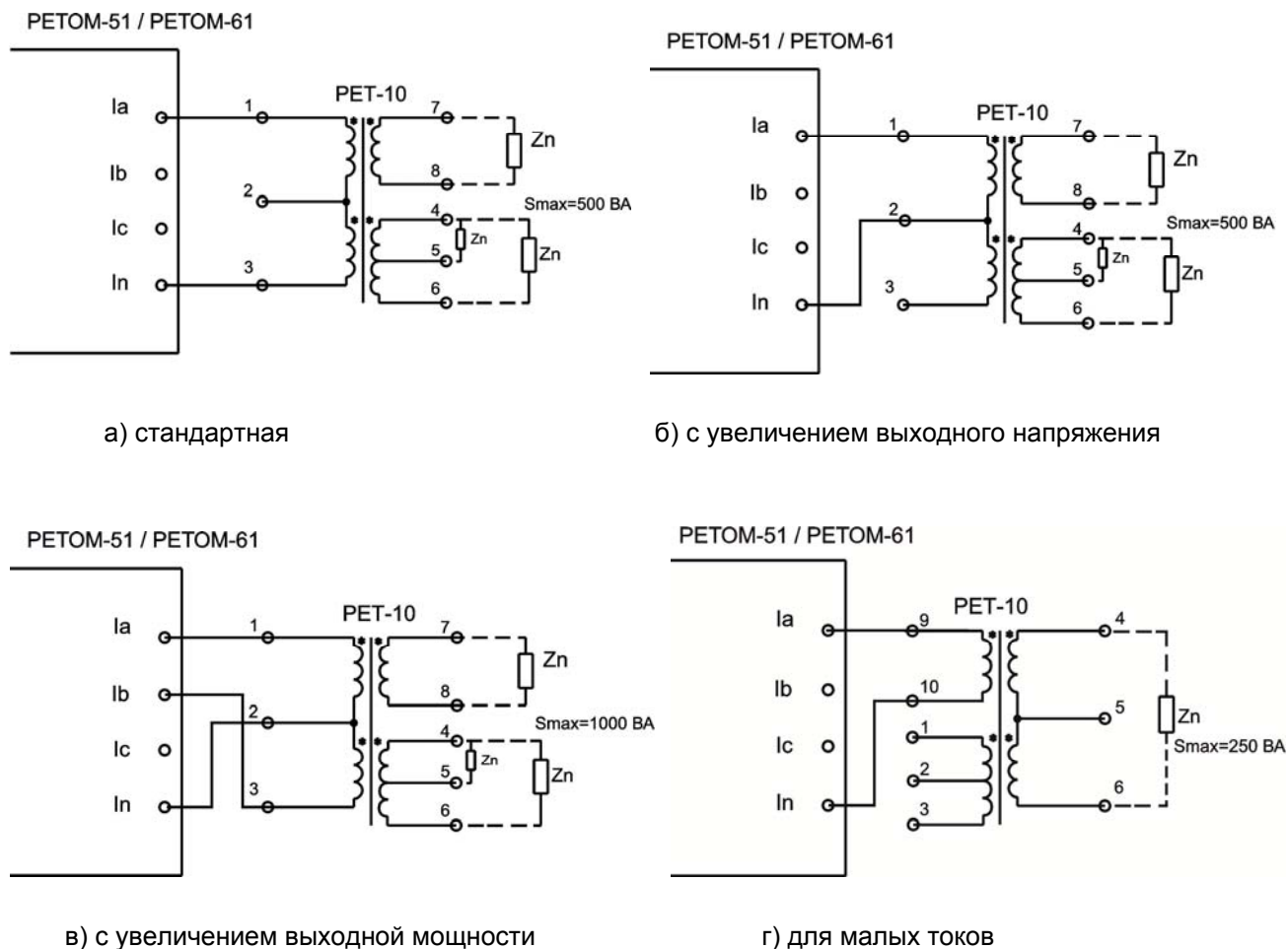
Рисунок 13.3 – Схемы подключения блока PET-10 к устройству PETOM-61 (PETOM-51)
