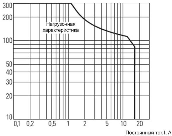
Рисунок 8.9 – Коммутационная способность выходных реле
