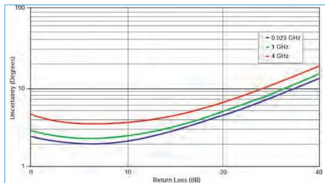
Погрешность фазы отраженного сигнала (S331D)
