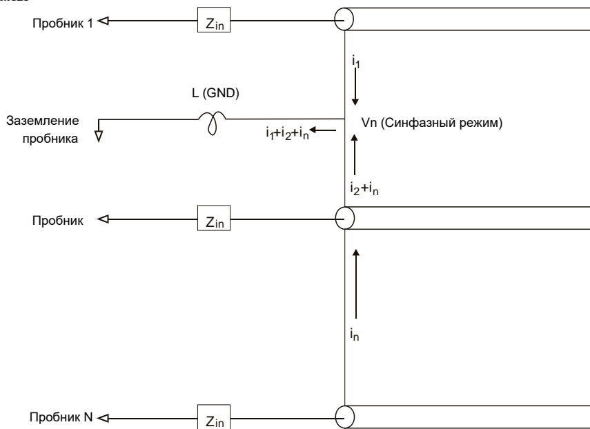
Рис. 25 Схема формирования синфазного входного напряжения. Помимо появления синфазного входного напряжения, длинный провод заземления ухудшает также точность воспроизведения формы импульсов в системе пробников. Увеличивается время нарастания и амплитуда "звона", обусловленного незадемпфированным LC-контуром на входе пробника. По-
