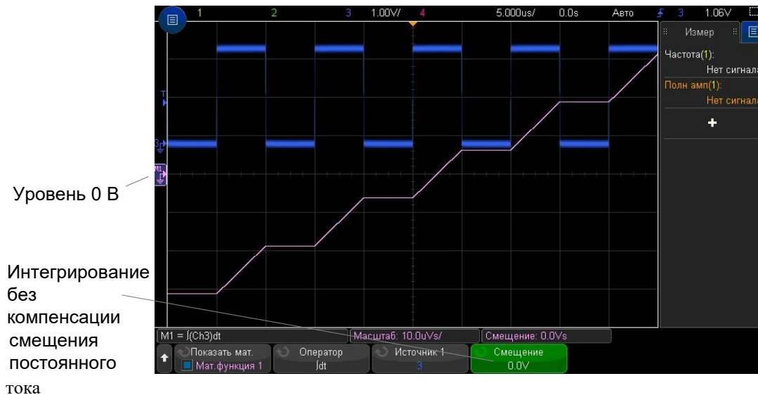
Рис. 9 Интегрирование без компенсации смещения постоянного тока
