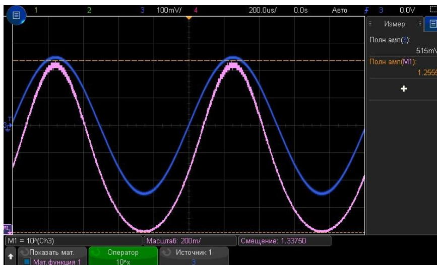
Рис. 15 Пример использования математической функции степени по основанию 10
