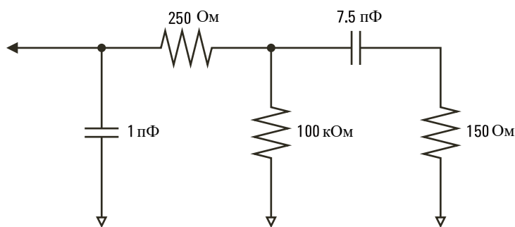
Рис. 22 Эквивалентная схема пробника для измерения напряжения постоянного тока и низкочастотного напряжения.
