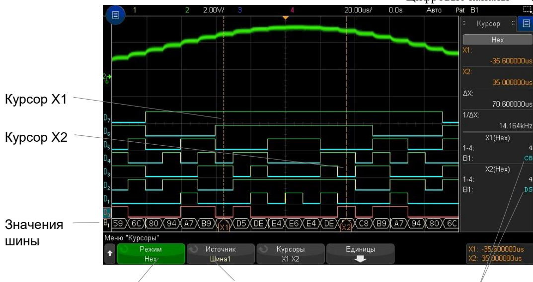
Установка для режима курсоров значения "Двоичный" или "Шестнадцатеричный" Выбор в качестве источника шины 1 или шины 2 Значения шины в местах курсоров, показанных здесь
