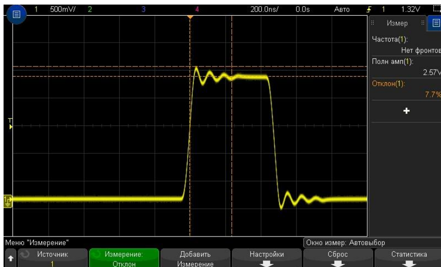
Рис. 48 Автоматическое измерение отклонения на вершине фронта
