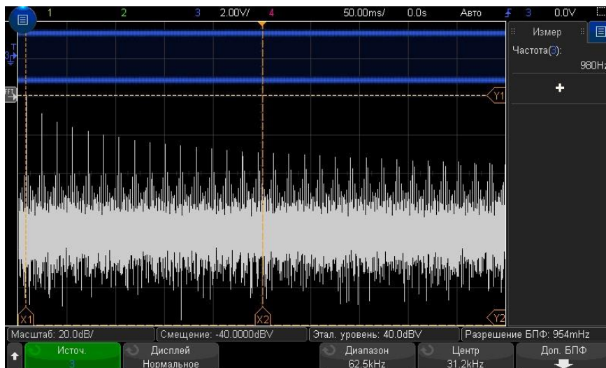
Рис. 5 Эффект наложения спектров
