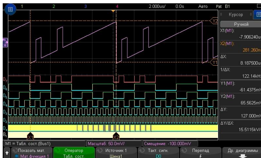
Рис. 20 Пример графика состояния логической шины
