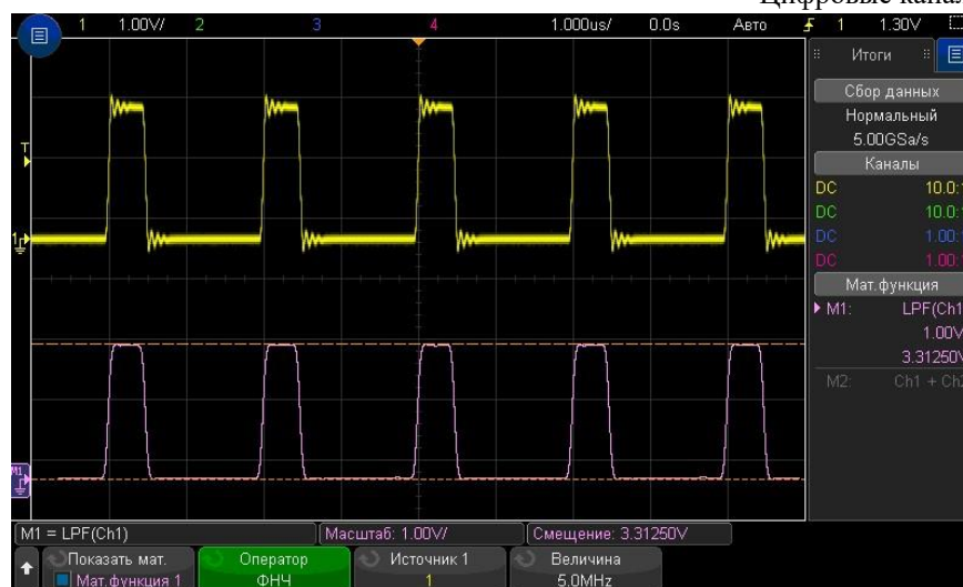
Рис. 16 Пример использования математической функции ФНЧ
