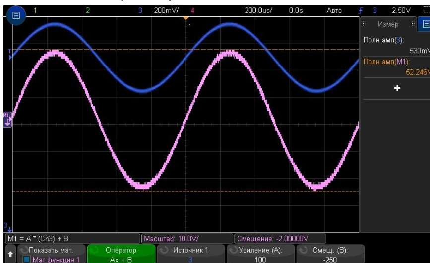
Рис. 12 Пример использования математической функции Ax + B
