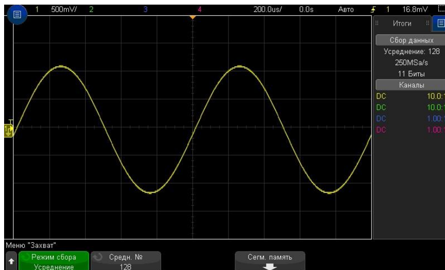
Рис. 40 Снижение уровня случайного шума при количестве усреднений 128.
