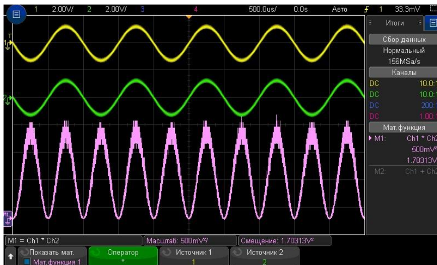
Рис. 7 Пример умножения сигнала канала 1 на сигнал канала 2
