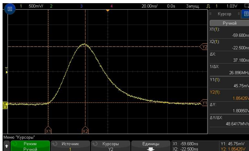
Рис. 41 Использование курсоров для измерения длительности импульса на произвольном уровне
