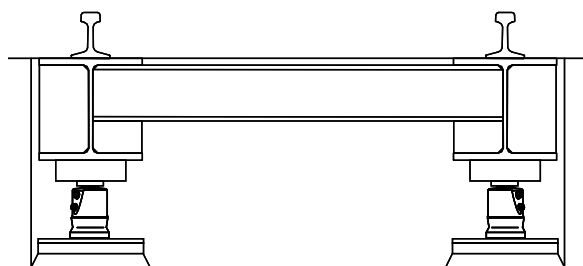
VRS241 в поперечном сечении
